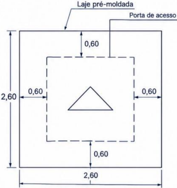
COBERTURA
