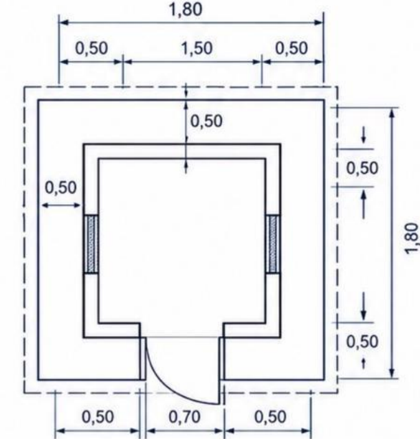
PLANTA BAIXA
