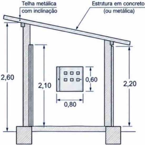
CORTE AB
