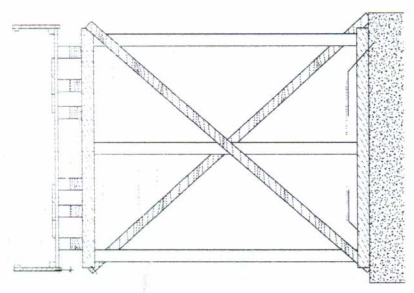
2 - CORTE AA Escala 1/40
